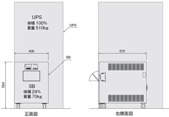
UPSとの寸法比較（SBシリーズ、10kVA）
