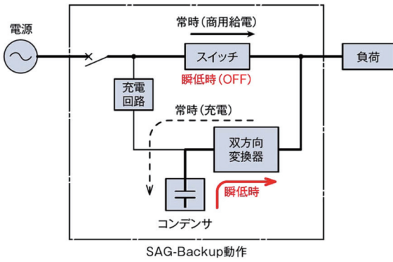
SBシリーズシステム構成
